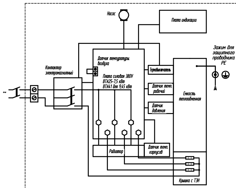
Рисунок 6. Схема подключения Wargmos-RX-7.5-9,45/220B
