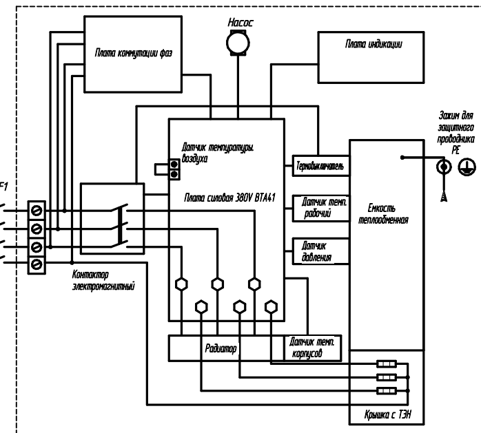
Рисунок 7. Схема подключения Wargmos-RX-7.5-18 (380B)
